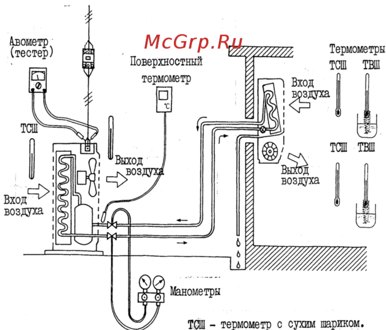
Рис. 8.1. Измеряемые параметры и применяемые приборы
