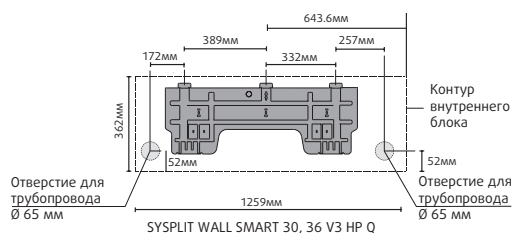
Табл. 2. Габариты внутреннего блока
