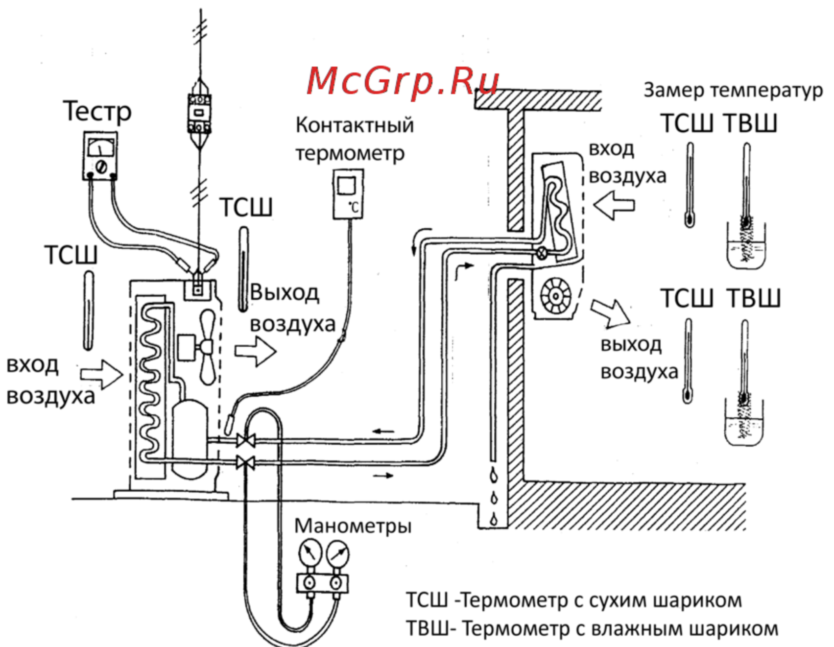
Рис. 8.1. Измеряемые параметры и применяемые приборы
